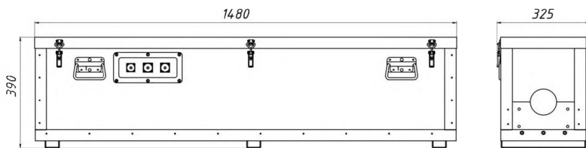
Алюминиевый ящик для плотногомера ПБ-В-75
